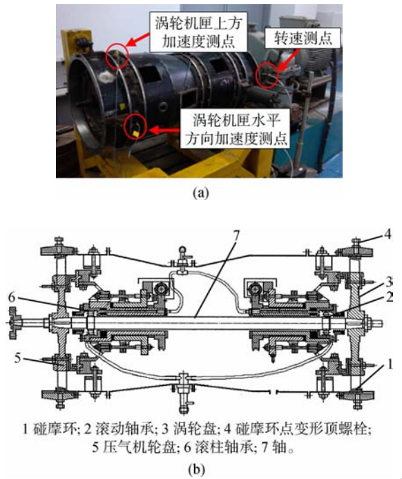
图 1 航空发动机转子试验器 Fig.1 Aero-engine rotor experimental rig
