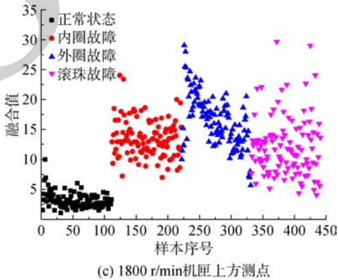
图 5 不同转速和测点下的融合结果 Fig. 5 Fusion results under different rotational speeds and measuring points
