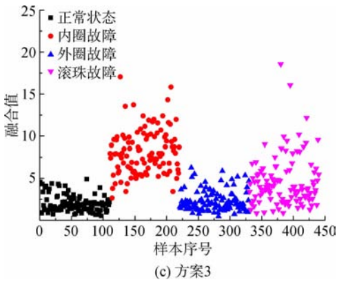
图 4 不同方案下的融合结果 Fig. 4 Fusion results under different schemes
