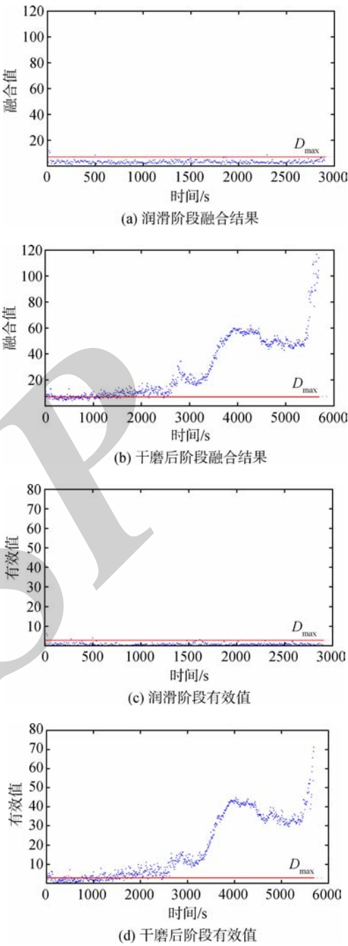
图 12 特征融合值与有效值对比
